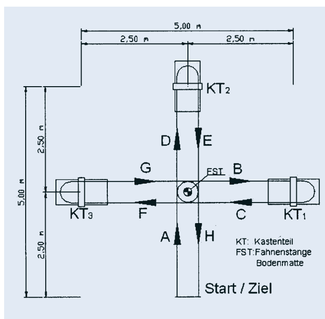
Abb. 3: Aufbauskeizze für den Hindernislauf
